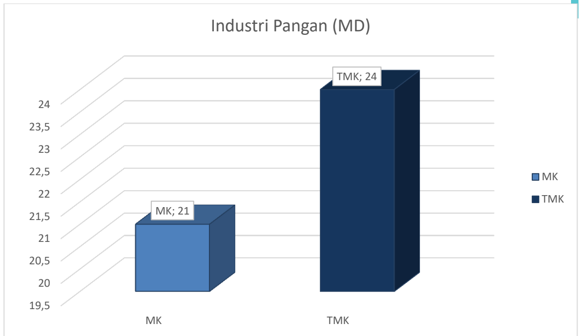
Gambar 15 Profil Hasil Pemeriksaan Industri Pangan Loka POM di Kabupaten Kediri
